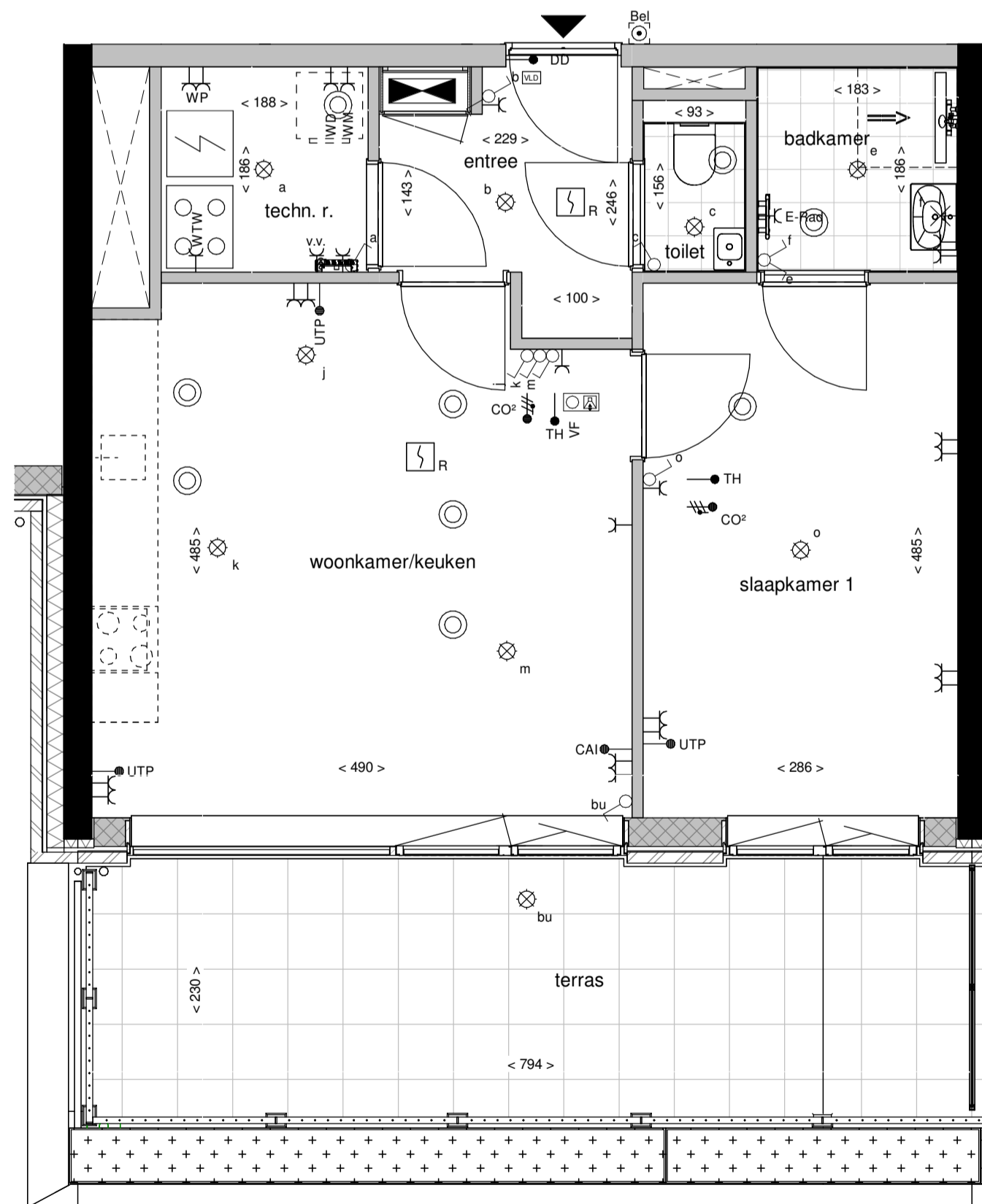
5e Verdieping
