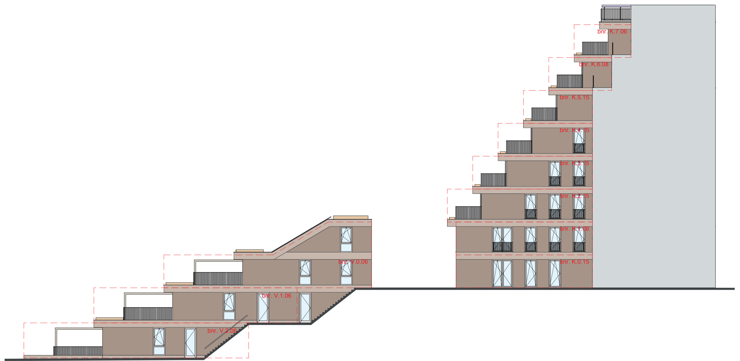
Oostgevel tussentrap
