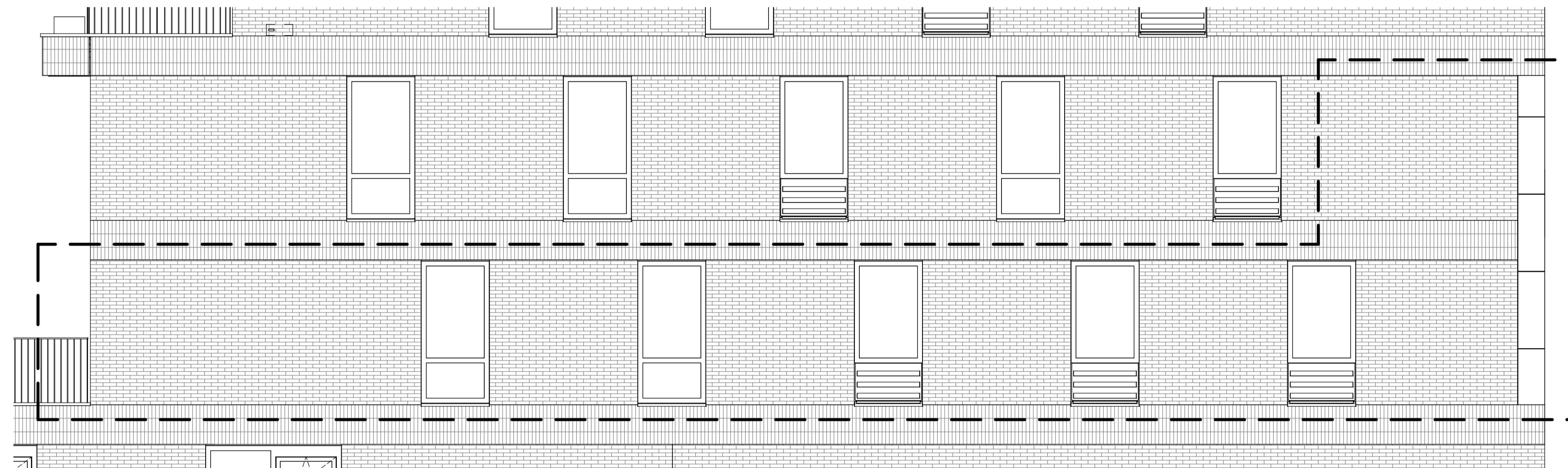
Zijgevel
