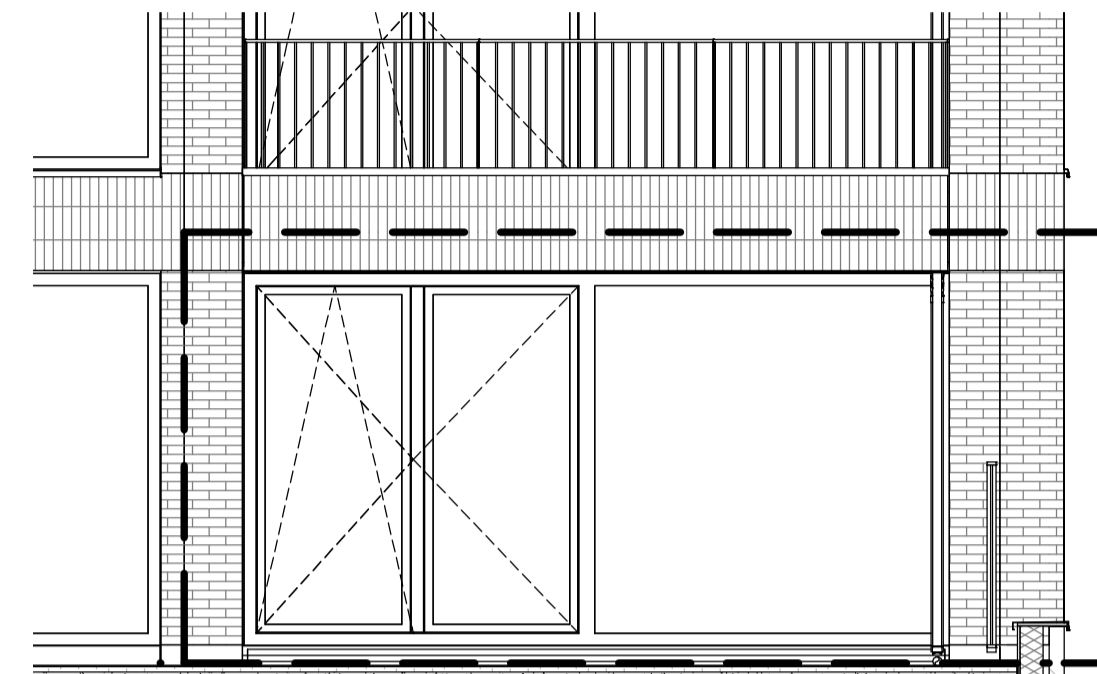
Voorgevel
