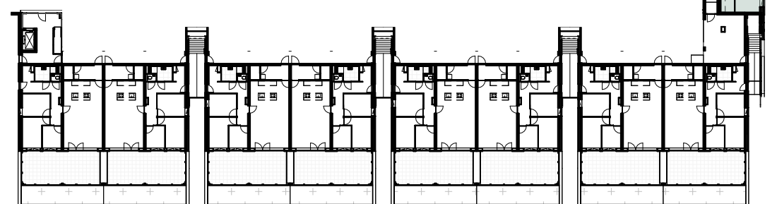
Overzicht, kelder -1
