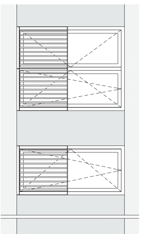
Zuidgevel
