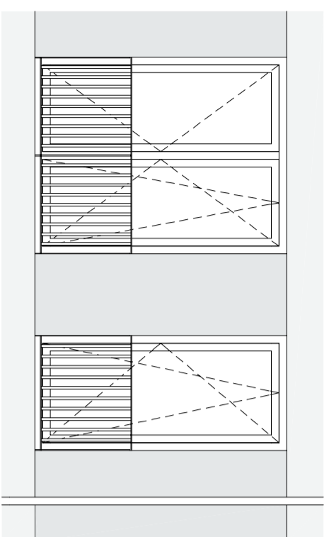
Zuidgevel
